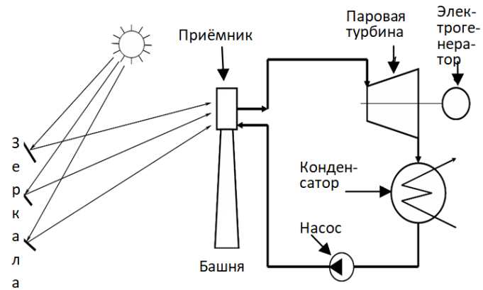
Рис. 2. Гелиотермальная электростанция
